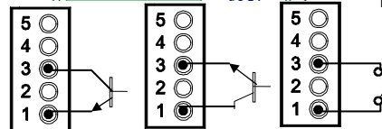
Fig. 20.2 Ejemplos de conexión. PNP, NPN o contacto libre.
