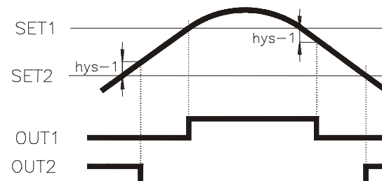
Actuación histéresis asimétrica
