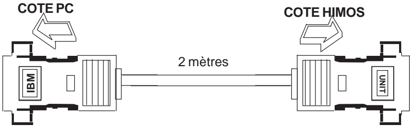
DB9 FEMELLE (RS232)
