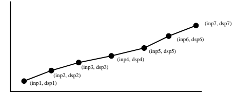
Fig. 17.1: Linealización por tramos. Ejemplo con 7 puntos y seis tramos.
