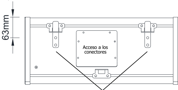
Vista posterior del visualizador con los soportes para su fijación.
